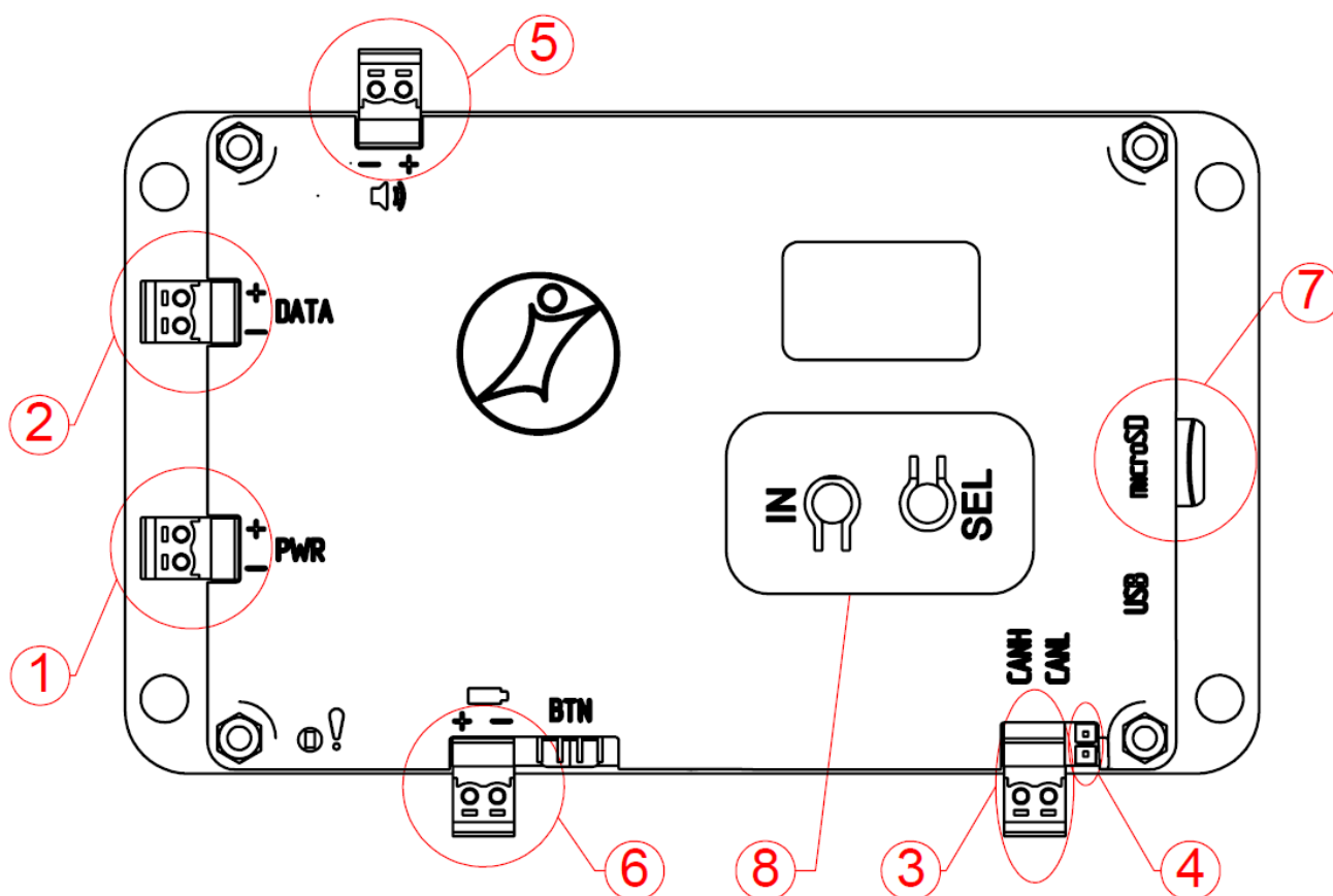
Рис.2. Основные разъемы и элементы управления устройства
